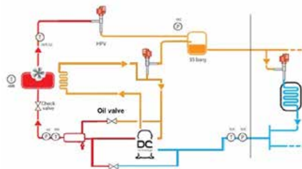
MODÈLE UMT T BTDX 2 - COMPRESSEUR BI-ÉTAGÉ
